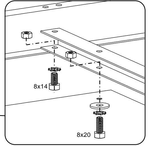
Universal Gehäuseunterbau 800-1200
