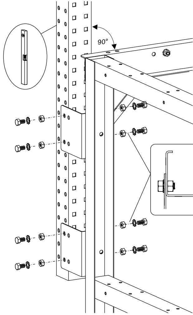
Aufbauportal Lochsäule an Universal-Standard
