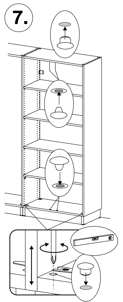
Sofort Anbauregal 50H
