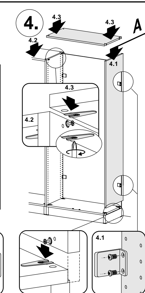
Sofort Anbauregal 50H
