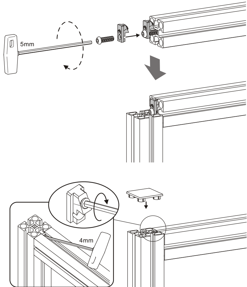
Aufbauportal Alu
