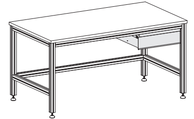
Einzelschukasten Alutisch 800
