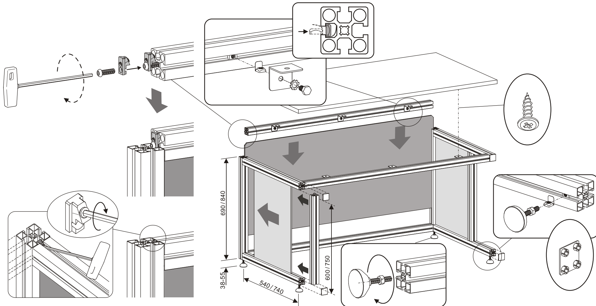
Alu-Pulttisch mit Sichtblende
